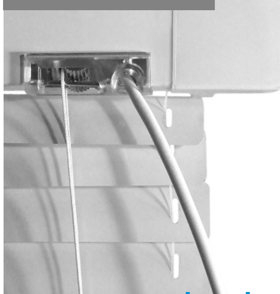
ISOLINE ECO: OVLÁDÁNÍ TYP2 BOVDEN + TYČKA
