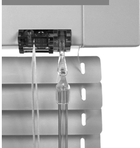
ISOLINE ECO: OVLÁDÁNÍ TYP1 ŠNEK + PLASTOVÉ TÁHLO
